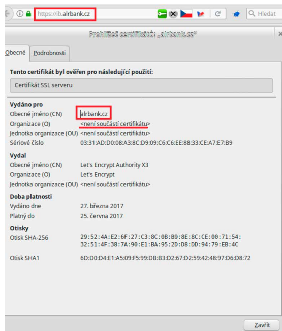
Obrázek 68: Falešný certifikát
