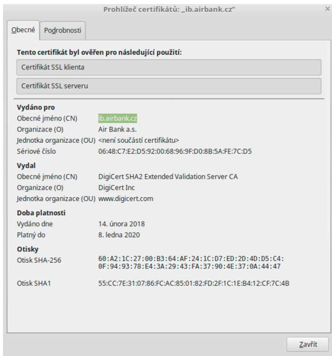
Obrázek 69: Pravý certifikát
