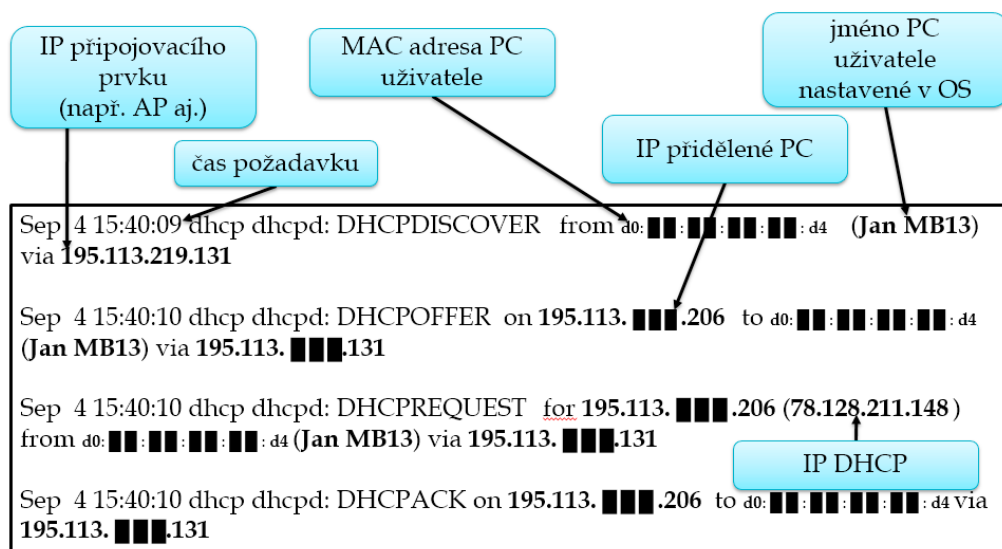
Obrázek 15: DHCP
